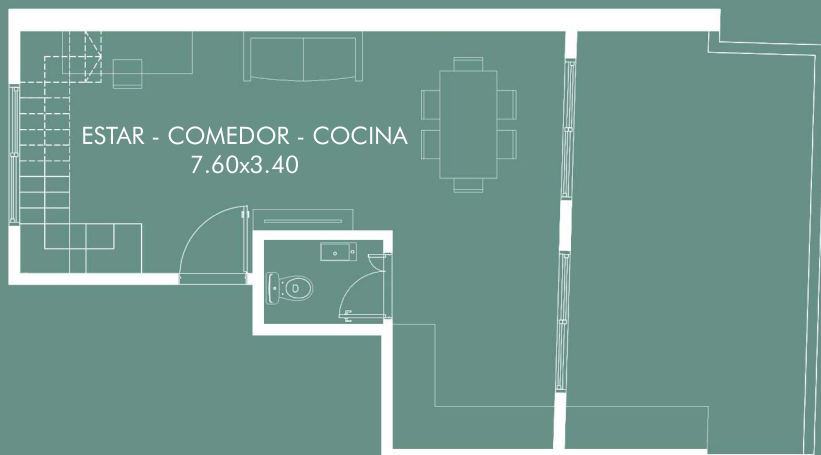
11° PISO
